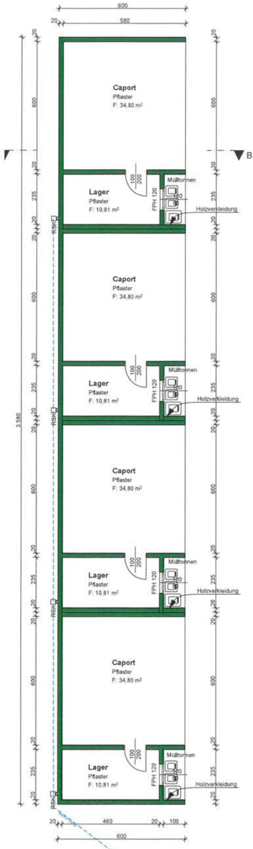
GRUNDRISS NEBENGEBAUDE
