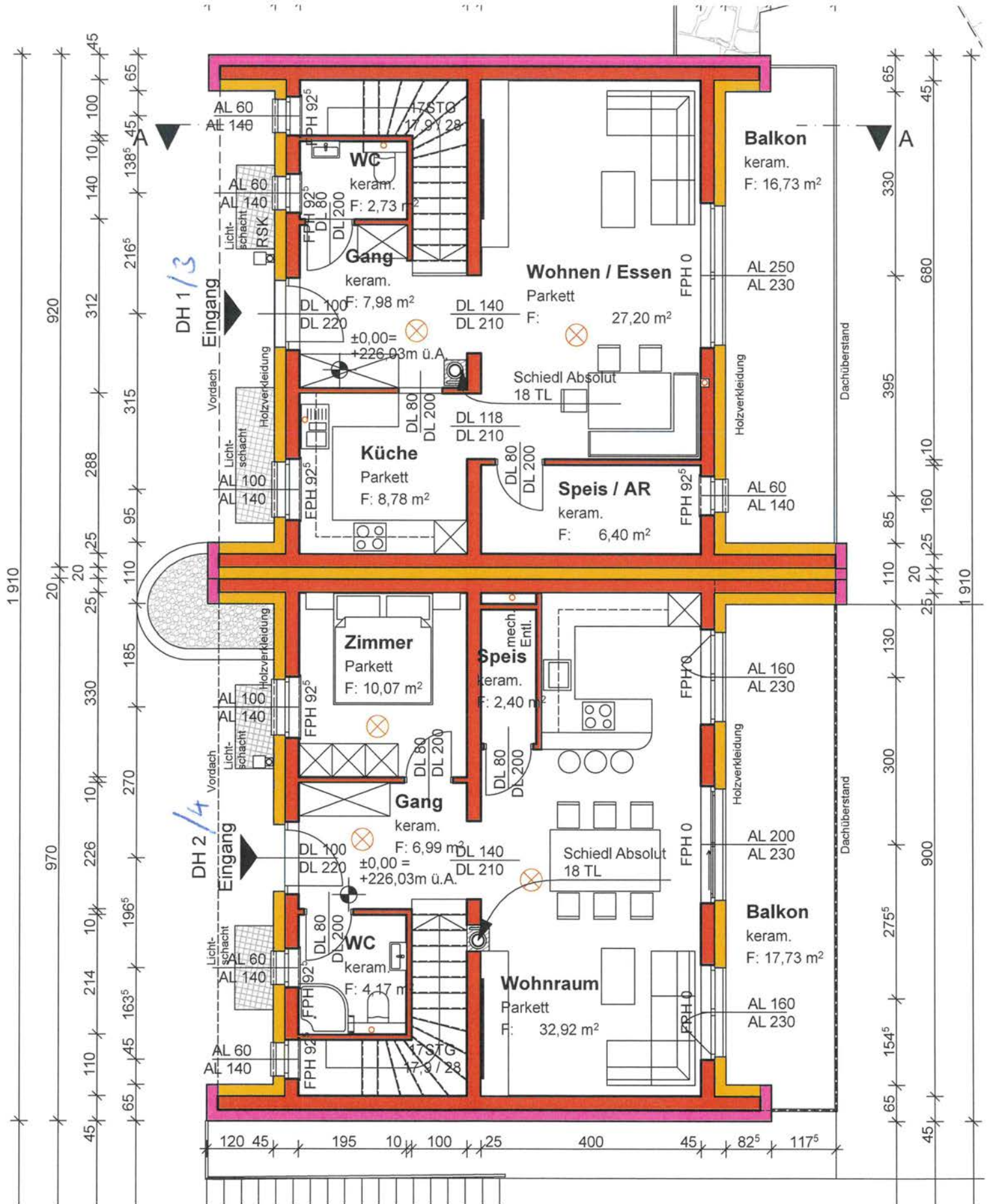
GRUNDRISS EG
