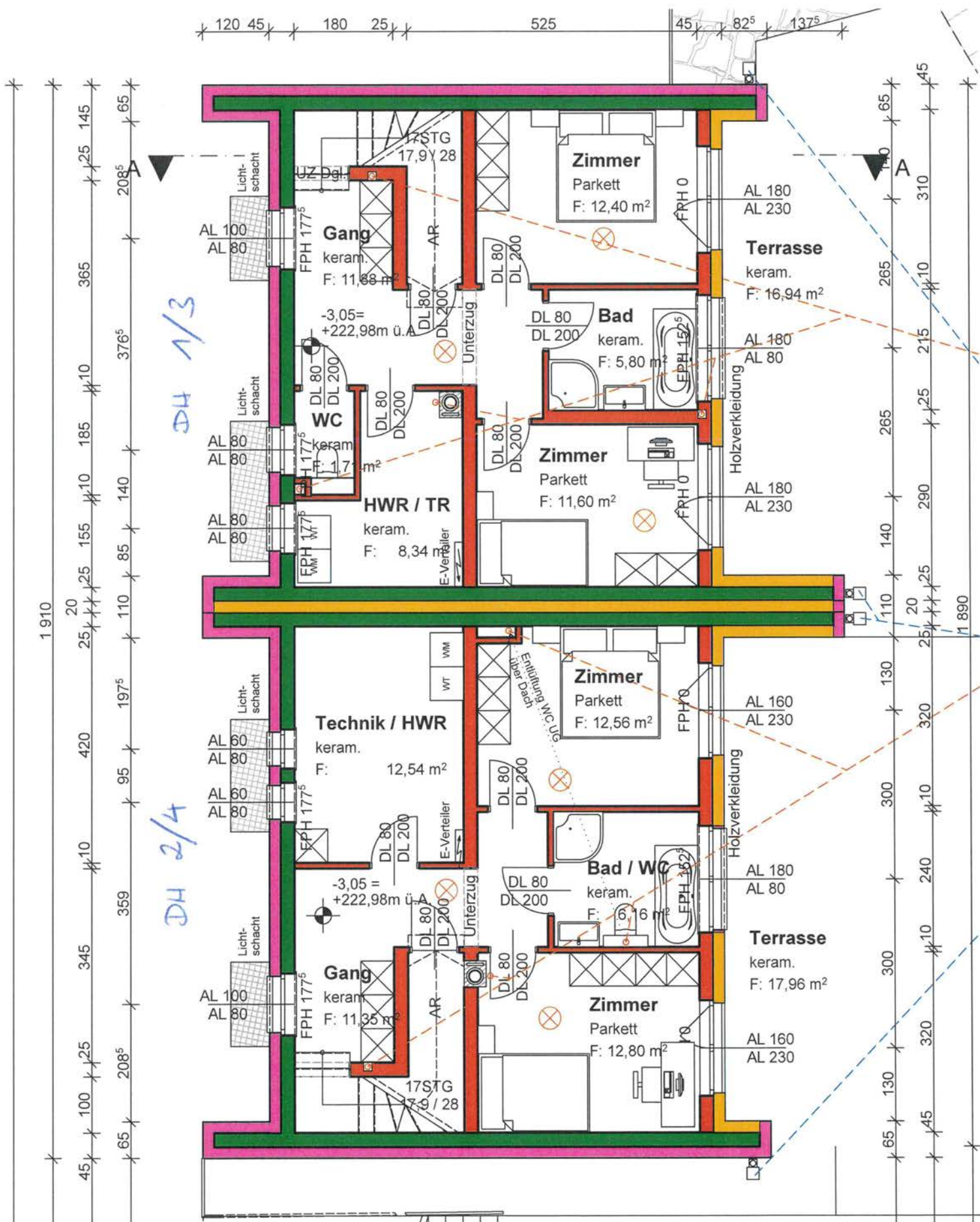
GRUNDRISS UG
