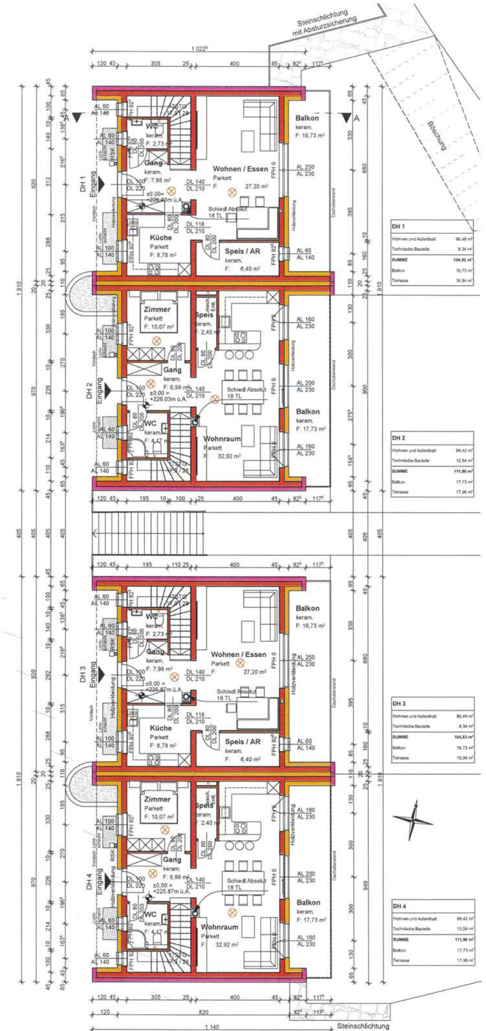
GRUNDRISS EG
